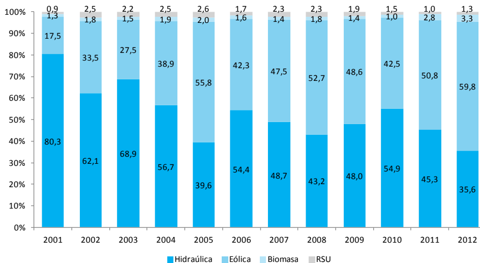
Gráfico 16. Estrutura da xeración eléctrica en Galicia
